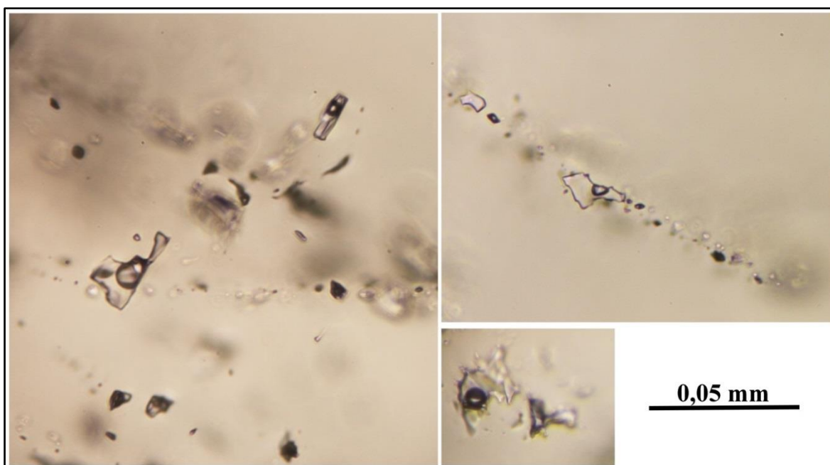
Slika 44. Fotografije fluidnih inkluzija u kvarcu, uzorak SA-18.
