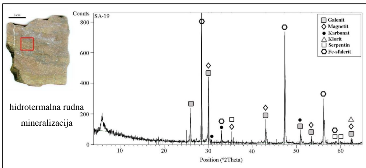
Slika 34. Rendgenogram uzorka SA-19.
