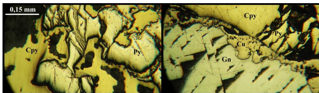
Slika 29. Mikrofotografija rudnih minerala u reflektiranom svjetlu, uzorak SA-24, vidljiva je zamjena pirita s halkopiritom; || polarizatori; (Cpy = halkopirit; Py = pirit; Gn = galenit; Cu = kuprit).
