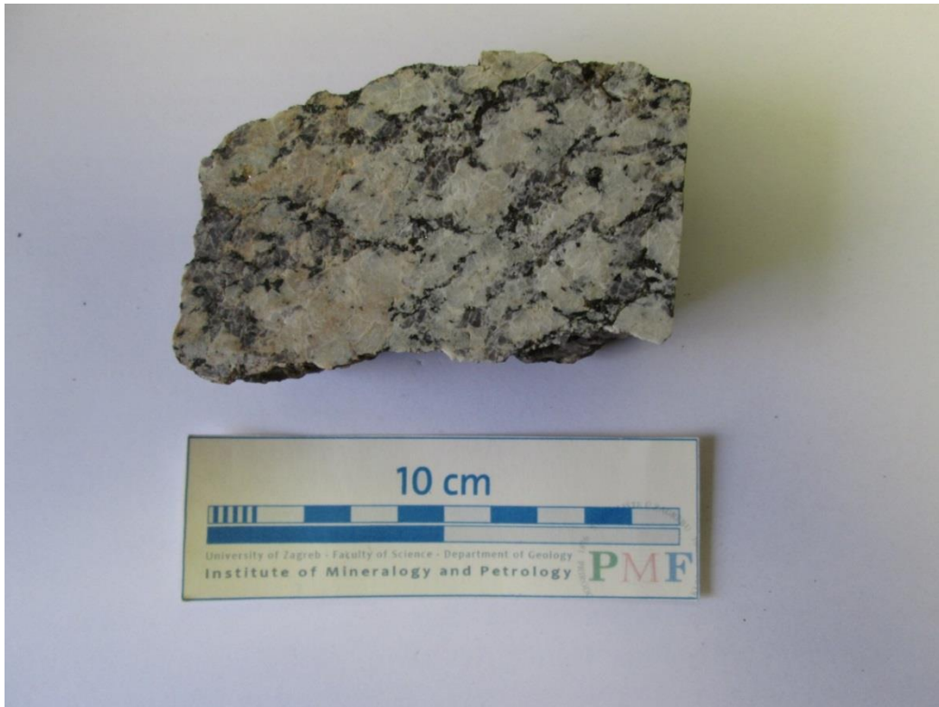
Slika 9 Makroskopski prikaz stijene s lokaliteta Koturić. Stijena je migmatit, vidno krupnozrnatija od granita sa istog područja.
