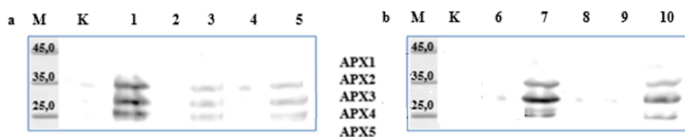
Slika 52. Imunodetekcija proteina APX u klijancima duhana koji su 30 dana rasli na podlogama koje su sadržavale a) AgNP i b) AgNO 3 . M – biljezi molekularskih masa (kDa), K – kontrola, 1 – 25 µM AgNP, 2 – 50 µM AgNP, 3 – 75 µM AgNP, 4 – 100 µM AgNP, 5 – 500 µM AgNP, 6 – 25 µM AgNO 3 , 7 – 50 µM AgNO 3 , 8 – 75 µM AgNO 3 , 9 – 100 µM AgNO 3 , 10 – 500 µM AgNO 3 .
