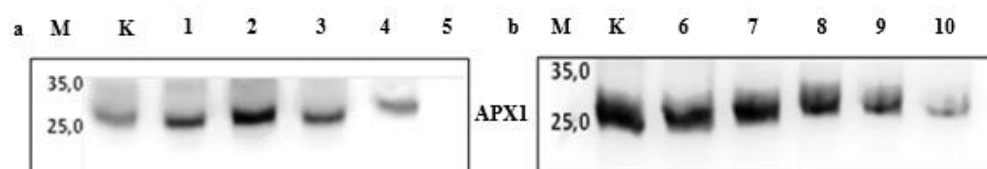
Slika 53. Imunodetekcija proteina APX u korijenu odraslih biljaka duhana koje su tretirane sedam dana u vodenim otopinama a) AgNP i b) AgNO 3 . M – biljezi molekularskih masa (kDa), K- kontrola, 1 – 25 µM AgNP, 2 – 50 µM AgNP, 3 – 75 µM AgNP, 4 – 100 µM AgNP, 5 – 500 µM AgNP, 6 – 25 µM AgNO 3 , 7 – 50 µM AgNO 3 , 8 – 75 µM AgNO 3 , 9 – 100 µM AgNO 3 , 10 – 500 µM AgNO 3 .
