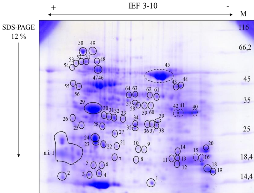
Slika 68. Ukupni topivi proteini klijanaca duhana tretiranih sa 100 \mu M \text{AgNO}_3 razdvojeni 2-DE. Gel je obojan bojom CBB i obrađen računalnim programom Image Master 2D Platinum . M – biljezi molekulske mase (kDa), IEF pI 3-10 – relativan položaj proteina na gelu u odnosu na vrijednost njihove izoelektrične točke, SDS-PAGE 12% – relativan položaj proteina na gelu u odnosu na njihove molekulske mase.
