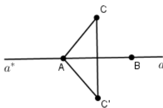
Slika 3.5: Dokaz Teorema 3.2.15
