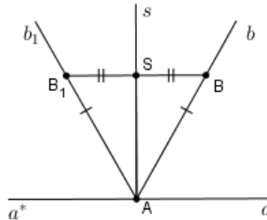
Slika 2.26: Dokaz Teorema 2.3.2 (2)
