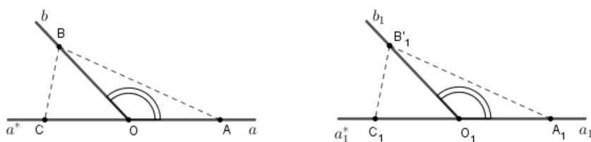
Slika 2.14: Dokaz Teorema 2.2.12
