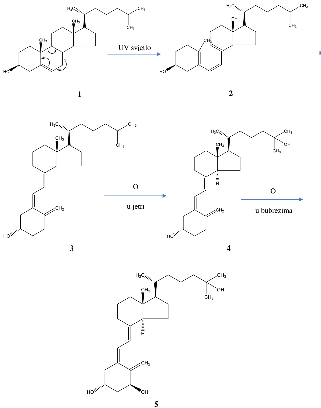
Slika 39. Prikaz sinteze vitamina D 3 ( 1 -7-dehidrokolesterol, 2 -provitamin D 3 , 3 -vitamin D 3 , 4 -kalsidiol, 5 -kalcitriol) 4
