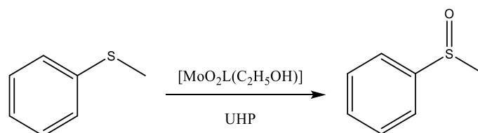
Slika 10. Shematski prikaz oksidacije sulfida uz katalizator [MoO 2 L(C 2 H 5 OH)], L = 2-N'-[1-(2-hidroksinaftil)etil]dien]-2-hidroksibenzoilhidrazon, UHP = kokristal tioureje i vodikovog peroksida 26
