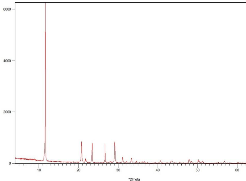
Slika 14. Difraktogram lake mineralne frakcije uzorka BG-Tuf III.
