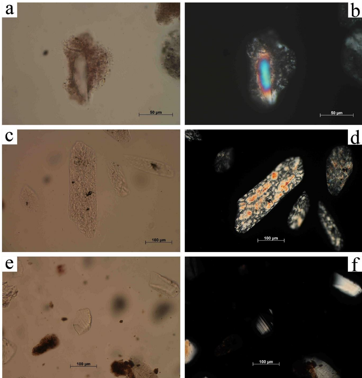
Slika 7. Fotografije mineralnih zrna iz uzoraka tufova: a, b - devitificirano staklo s kvarcom u središtu (BG-Tuf I); c, d - gips (BG-Tuf III); e, f - plagioklas (BG-Tuf IV).
