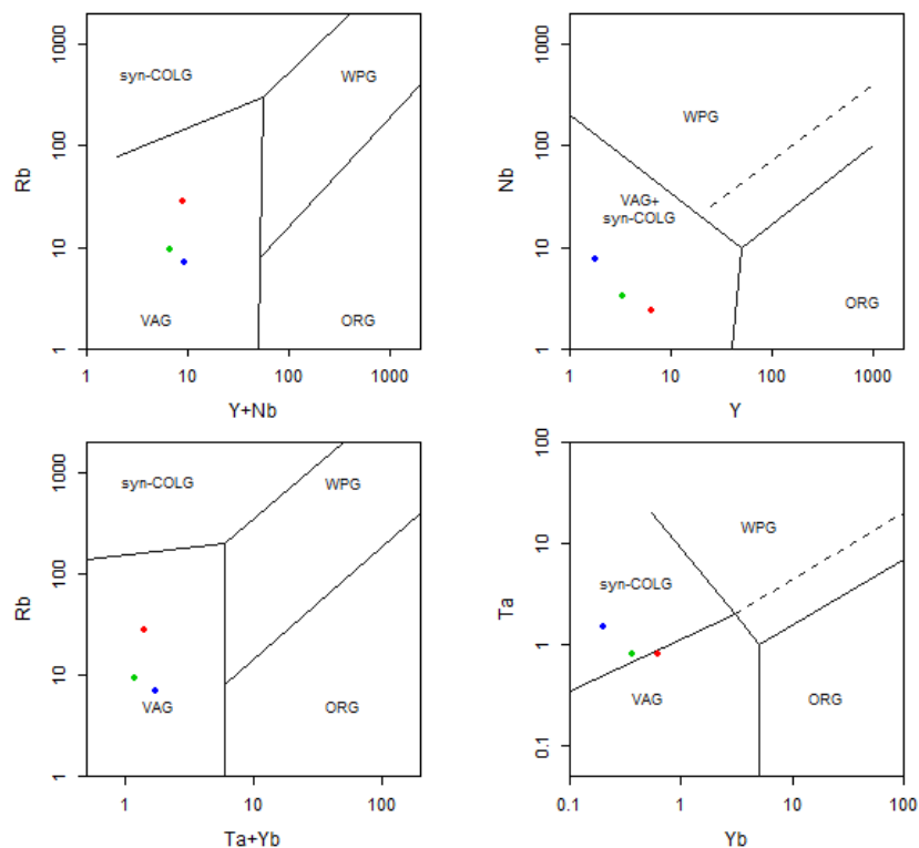
Slika 26. Dijagrami za geotektonski smještaj kiselih vulkanskih stijena prema Pearce i dr. (1984). Kružni oblici označavaju pojedine uzorka tufova: crvena - BG-Tuf I; zelena - BG-Tuf III; plava - BG-Tuf IV. ORG - graniti oceanskih hrptova ( ocean ridge granites ); VAG - graniti vulkanskih lukova ( volcanic-arc granites ); WPG - graniti smješteni unutar ploče ( within-plate granites ); syn-COLG - sin-kolizijski graniti ( syn-collisional granites ).
