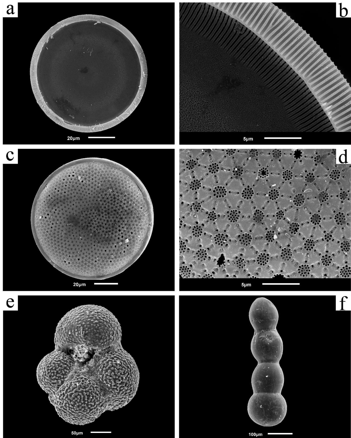
Slika 19. SEM fotografije fosilnog sadržaja. a) i c) dijatomeja (BG-Tuf IV P); b) i d) detalj dijatomeje (BG-Tuf IV P); e) Globigerina bulloides d'Orbigny, 1826 (BG-Tuf IV K); f) Orthomorphina dina (Venglinški, 1958) (BG-Tuf IV K).
