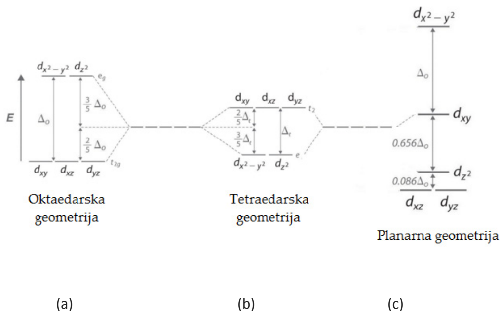
Slika 2.1. Cijepanje ligandnog polja za (a) oktaedarski, (b) tetraedarski i (c) kvadratno koordinirane komplekse.
