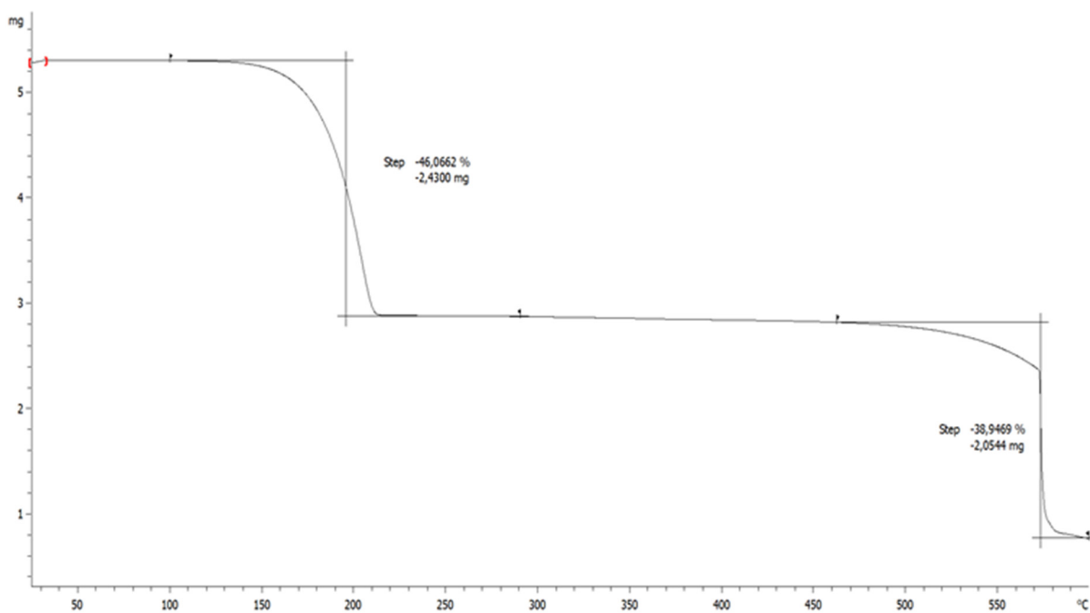
Slika D19. Termogravimetrijska krivulja spoja [\text{CdBr}_2(2\text{-Clpz})_2]_n (4)
