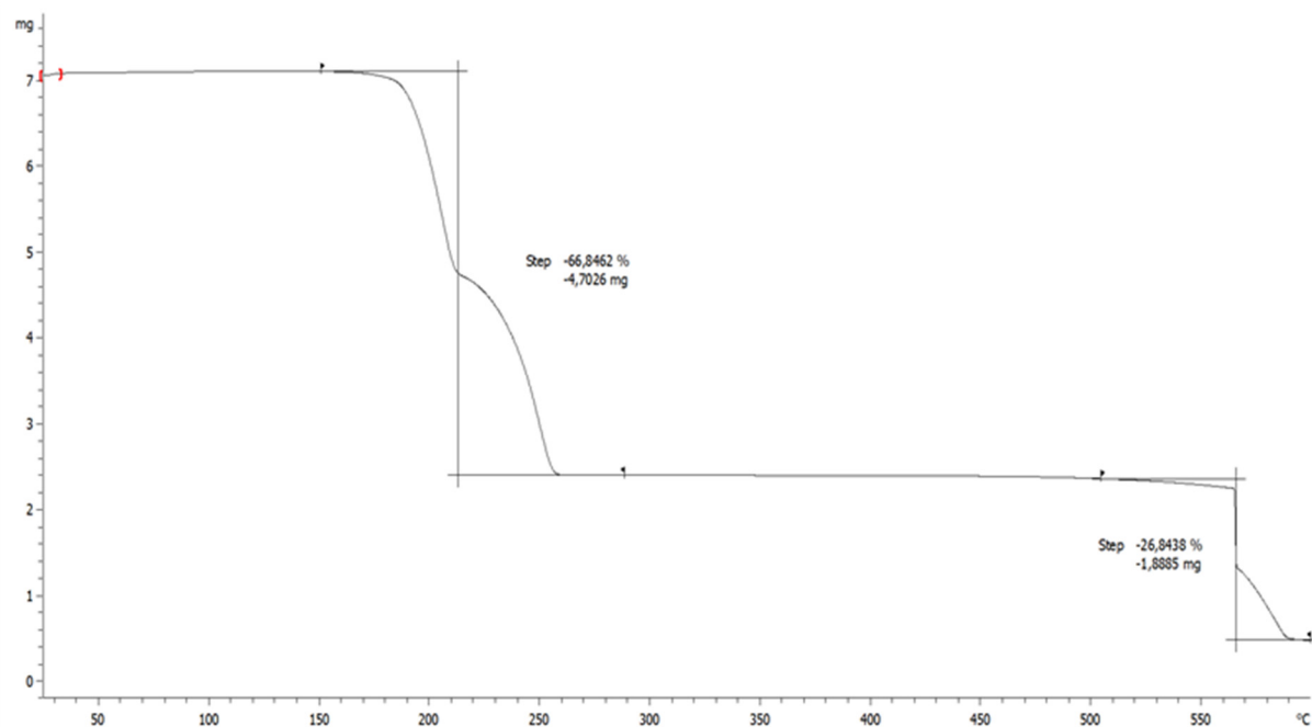
Slika D18. Termogravimetrijska krivulja spoja [\text{CdCl}_2(2\text{-IPz})_2]_n (3)
