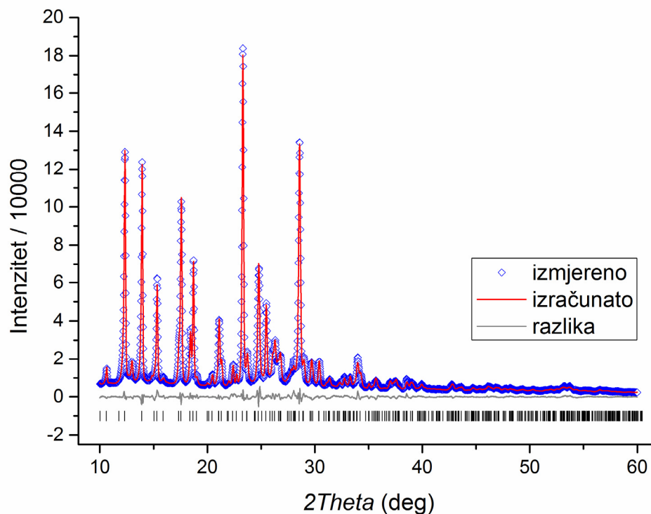
Slika 32. Rietveld utočnjavanje izmjerene i izračunate difraktograma za strukturu kokristala 9-mG:1-mC. Ispod 2\theta = 10^\circ nema difrakcijskim maksimuma. Izračunati položaji difrakcijskih maksimuma označeni su vertikalnim crticama.
