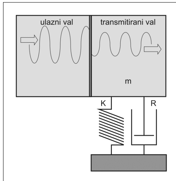
Slika 4.1. Shematski prikaz prijenosa energije s jednog harmoničkog oscilatora na drugi. Zbog trenja u sustavu dio energije vala se pretvara u toplinu.
