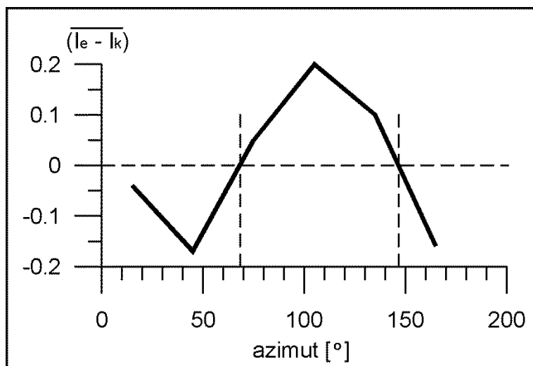
Slika 3.4. Azimutalna ovisnost srednjih razlika empirijskih intenziteta i intenziteta izračunatih za izotropni model. Vrijednosti su računane za klase širine 30°.
