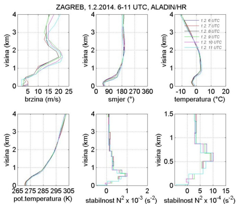
Slika 5.14. Vertikalni profil brzine vjetra (m/s, gore lijevo), smjera vjetra ( ^{\circ} , gore sredina), temperature zraka ( ^{\circ}\text{C} , gore desno), potencijalne temperature (K, dolje lijevo), kvadrata uzgonske frekvencije ( \text{s}^{-2} , dolje sredina) i uvećani profil kvadrata uzgonske frekvencije ( \text{s}^{-2} , dolje desno) za Zagreb za 1.2.2014. u 0–5 UTC (gore) i 6–11 UTC (dolje) prema pseudotempovima dobivenih modelom ALADIN/HR.
