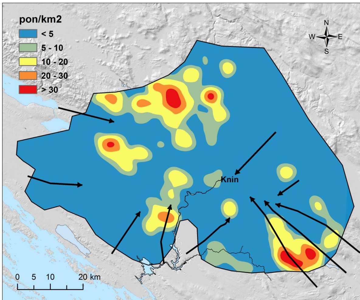
Slika 19. Gustoća ponikava
