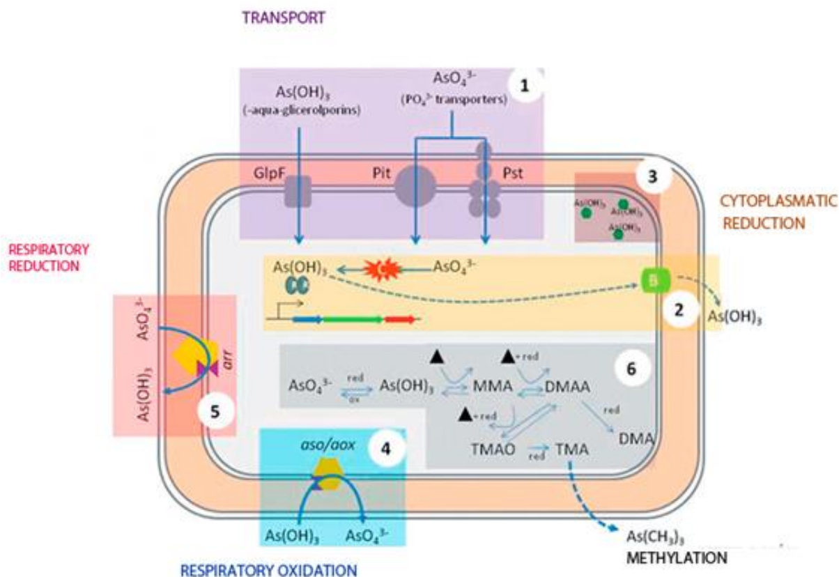
Slika 3. Glavni mehanizmi prokariotske rezistencije na arsen. 1) Arsenat ulazi u stanicu kroz fosfatne kanale dok arsenit ulazi kroz akvagliceroporine (2) Arsenat se reducira do arsenita
