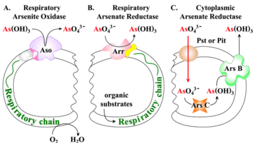
Slika 5. Stanična lokacija i funkcija bakterijske arsenit-oksidaze, respiratorne arsenat-reduktaze i citoplazmatske arsenat-reduktaze. A) Arsenit-oksidaza sudjeluje u oksidaciji arsenita u manje toksičan oblik, arsenat. B) Respiratorna arsenat-reduktaza reducira arsenat u arsenit. C) Citoplazmatska arsenat-reduktaza u citosolu reducira arsenat u arsenit pomoću ArsC, a nastali arsenit se izbacuje iz stanice pomoću ArsB. Preuzeto iz [17].
