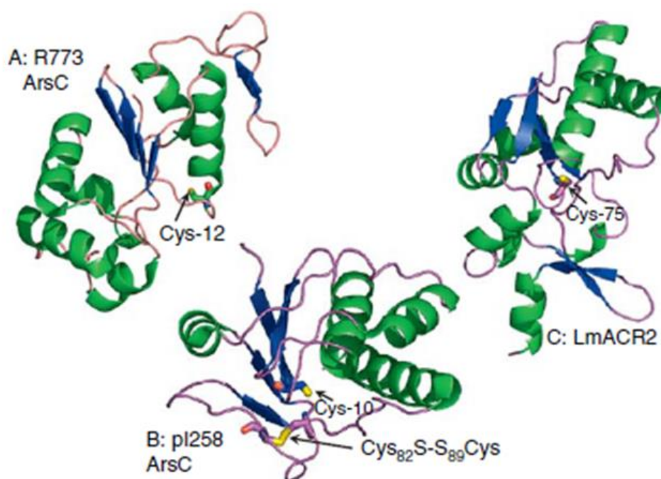
Slika 6. Struktura arsenat-reduktaze. A) i B) Sekundarna struktura ArsC na plazmidu R773 i pl258 sadrži katalitičke cisteine u aktivnim mjestima. C) Sekundarna struktura ArsC kod bakterije Leishmania LmACR2, koja ima slično aktivno mjesto kao i ljudski protein Cdc25a. Preuzeto iz [6].
