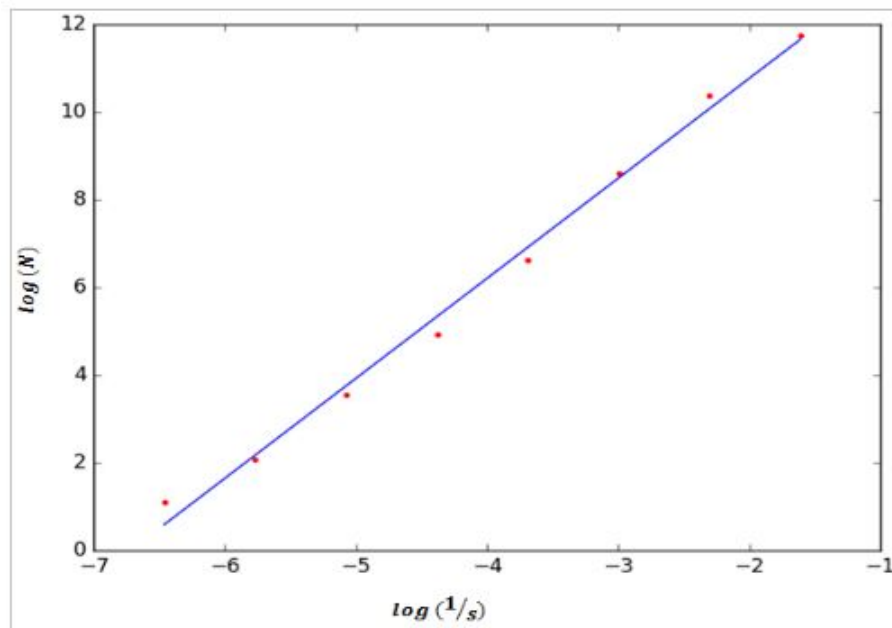
Slika 3.4: Pramac linearne regresije za profil Jamskog sustava Kita Gaćešina – Draženova puhaljka (za 3000 točaka)
