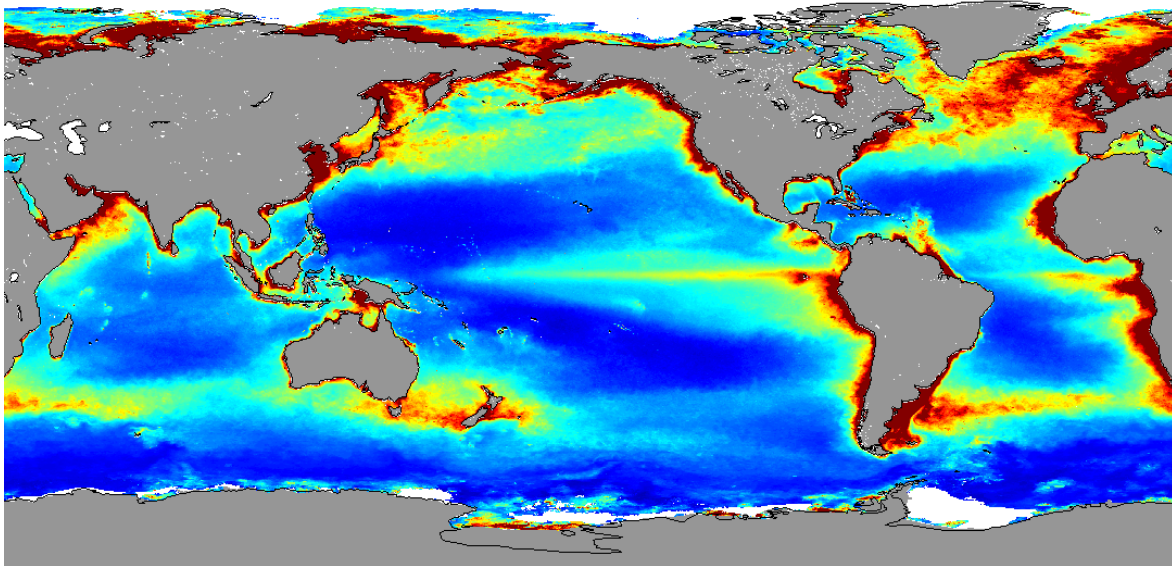
Slika 9. Globalna oceanska primarna proizvodnja (fotosinteza); Preuzeto iz http://www.science.oregonstate.edu/ocean.productivity/custom.php
