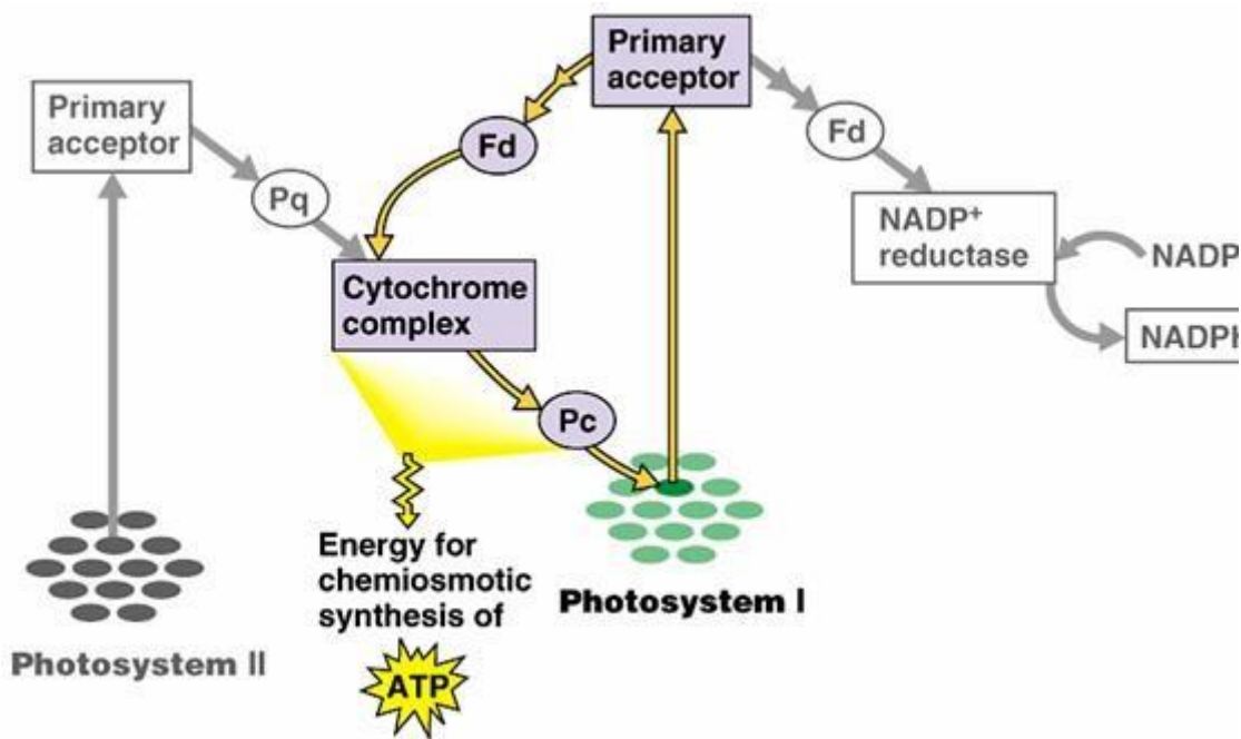
Slika 3. Prikaz fotosistema I i II povezanih transportnim lancem elektrona;Preuzeto iz
