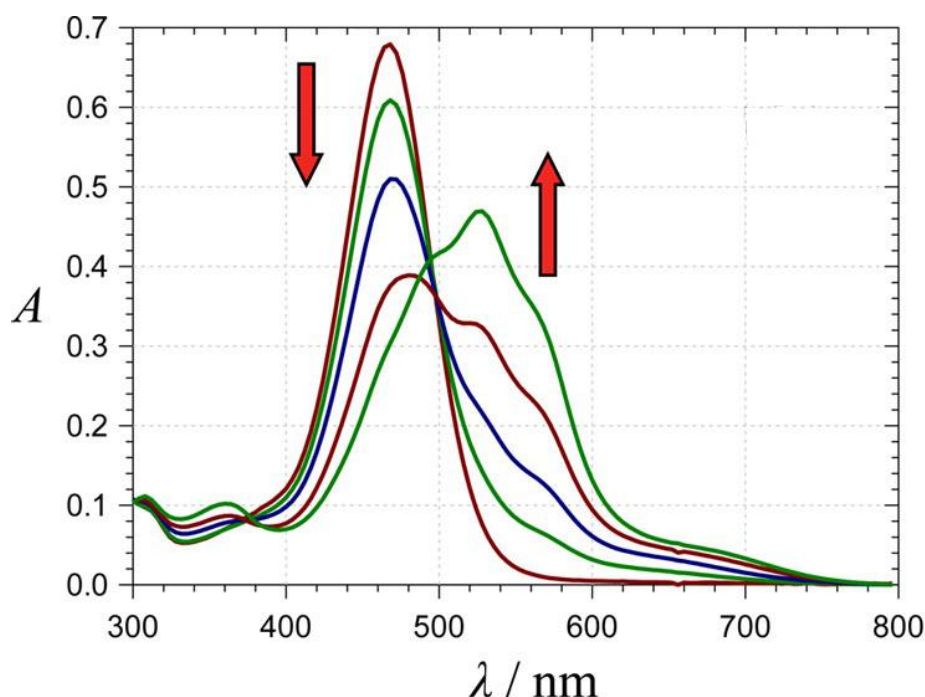
Slika 17: Ovisnost apsorbancije o valnoj duljini prilikom reakcije brzog nastajanja neutralne ( A ) i anionske forme ( A^- ) analoga antocijanina tijekom njegova dodavanja u pufer ( \text{pH} = 2 \rightarrow \text{pH} = 6 ) 1
