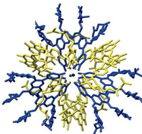
Slika 19: Kristalna struktura protocijanina dobivena difrakcijom rendgenskog zračenja 16
