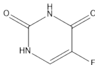
Slika 20. Struktura 5-Fluorouracila
