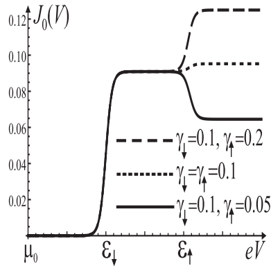
Slika 3.2: Prikazana je strujno - naponska karakteristika za nekoliko odabira magnetoskog mikrokontakta D, dok je iscrtkano prikazana za normalni metalni mikrokontakt. Pritom je J_0 u e\Gamma jedinicama, a temperatura je k_B T = 0.04|\epsilon_\uparrow - \epsilon_\downarrow| [3].
