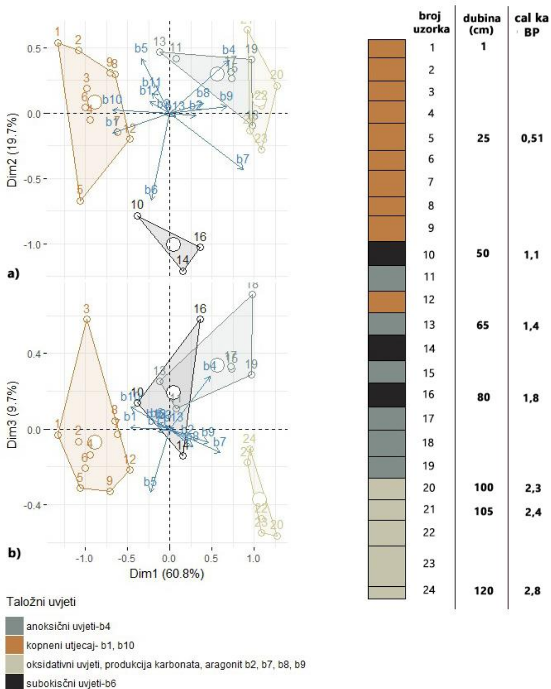
Slika 53 Prikaz analize glavnih komponenti (PCA) za marinski okoliš jezgre M1-A, a) u ravni Dim 1 i Dim 2 te b) u ravni Dim 1 i Dim 3. Vidljivo je grupiranje uzoraka ovisno o utjecaju pojedinih balansa odnosno geokemijskih specifičnosti. U drugom dijelu slike prikazana je rekonstrukcija jezgre ovisno o pripadnosti pojedinog uzorka određenoj grupi s okvirnim kronološkim okvirom temeljenim na modelu dubina starost za jezgru M1-A.
