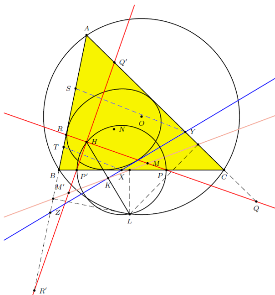
Slika 4.1: Droz-Farnyjeva anvelopa
