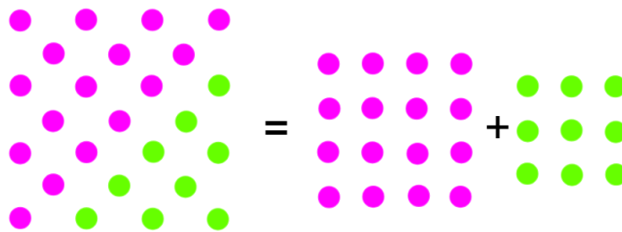
Slika 1.19: Geometrijski prikaz propozicije 1.24 za n = 4
