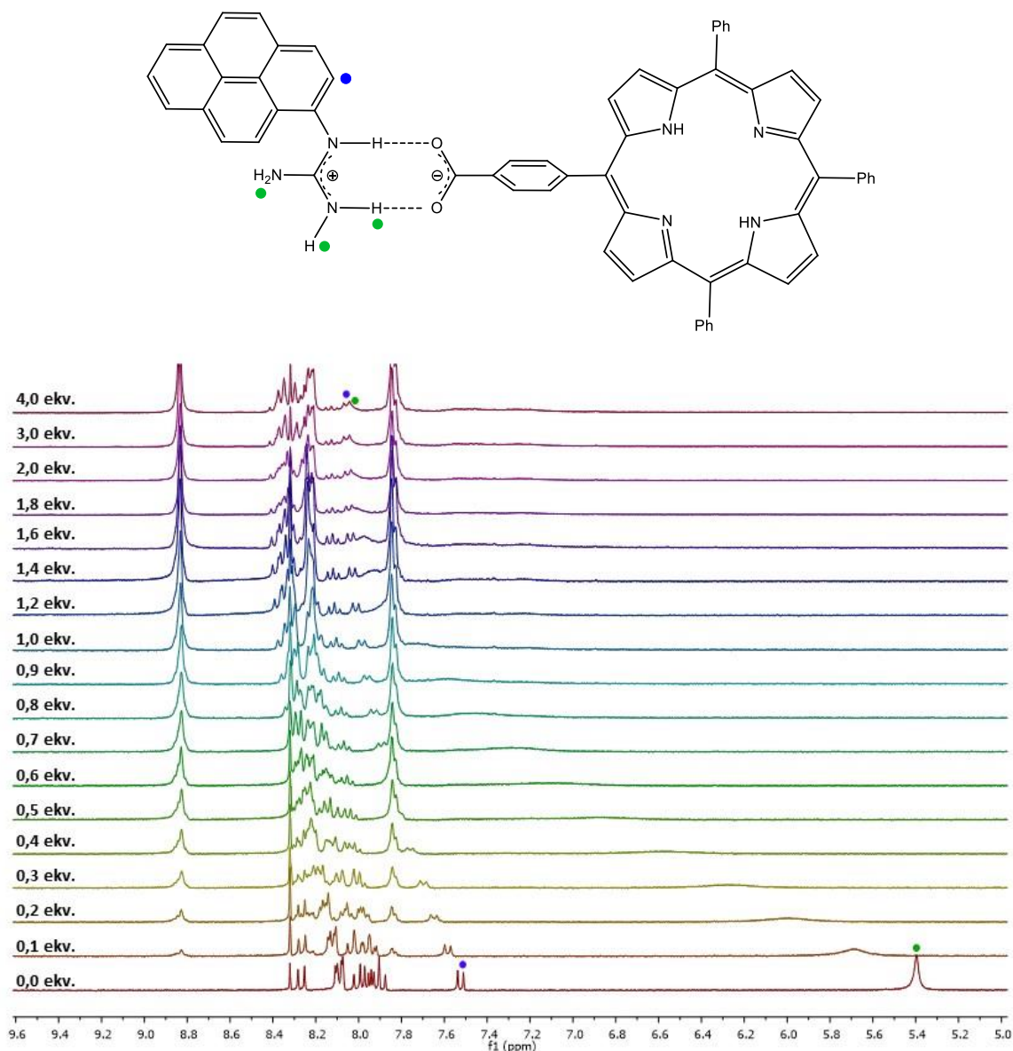
Slika 57. 1 H NMR titracija 16 ( 2,0 \times 10^{-3} mol dm -3 ) s 22 od 0 do 8,0 \times 10^{-3} mol dm -3 (4,0 ekvivalenta) u d 6 -DMSO pri 25°C.
