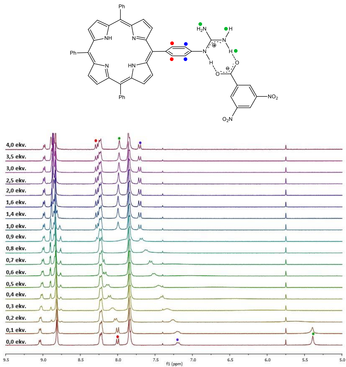
Slika 45. 1 H NMR titracija 20 ( 2,0 \times 10^{-3} mol dm -3 ) s 3,5-DNBA od 0 do 8,0 \times 10^{-3} mol dm -3 (4,0 ekvivalenta) u d 6 -DMSO pri 25°C.
