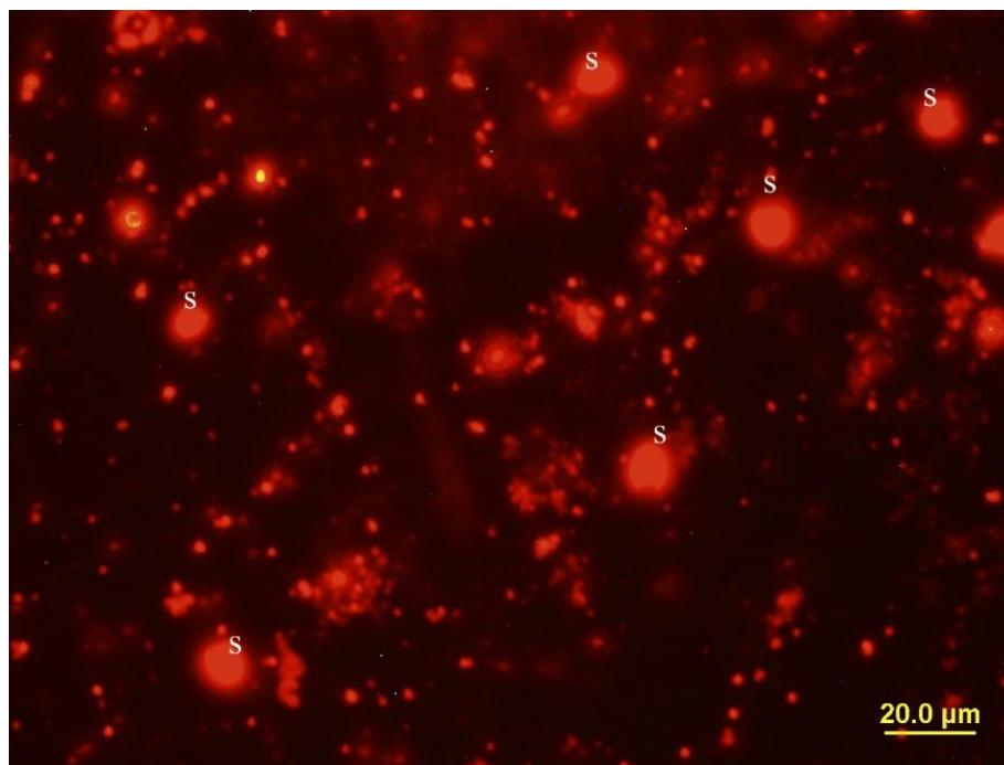
Slika 13. Fluorescentna mikrografija u kulturi stanica u prisutnosti kadmija koncentracija 1000 \mu g/L te uz Nile Red bojanje. s-stanice.
