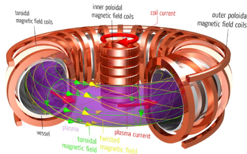
Slika 2.2: Princip rada tokamak uređaja [7]
