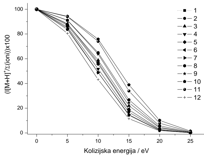
Dodatak 8.18. Omjeri relativnih intenziteta signala protoniranih hidrazona i svih iona u ovisnosti o kolizijskoj energiji.
