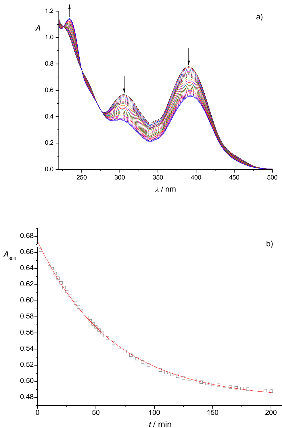
Dodatak 8.119. a) UV spektri spoja 10 u sustavu otapala metanol/vodi 1/1. Prvi spektar snimljen je dvije minute nakon pripreve otopine, dok su ostali snimani svake 4 minute kroz 180 minuta: c(\mathbf{10}) = 5 \times 10^{-5} \text{ mol dm}^{-3} , c(\text{OH}^-) = 0,10 \text{ mol dm}^{-3} , I_c = 1 \text{ mol dm}^{-3} (NaCl), l = 1 \text{ cm} , \theta = (25,0 \pm 0,1) \text{ }^\circ\text{C} . b) Vremenska ovisnost apsorbancija pri 304 nm.
