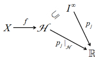
Slika 6.1: f neprekidna \Rightarrow p_j \circ f neprekidna.
