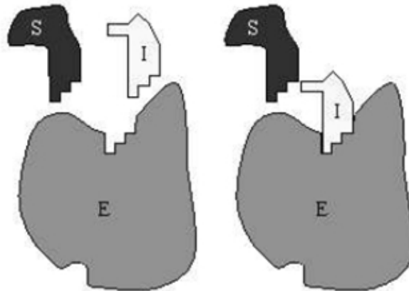
Slika 3.4: Kompetitivna inhibicija
