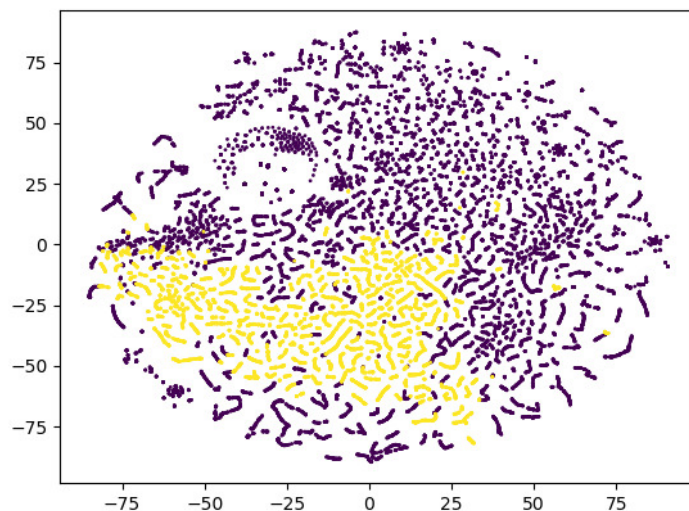
Slika 4.10: Vizualizacija klasteriranja pomoću autoenkodera i TSNE algoritima. Žutom bojom su označena područja koja reprezentiraju zadatak, a ljubičastom nagradu. Vidimo da možemo odvojiti stanja nagrade i zadatka, iako granica možda nije strogo definirana. Međutim, algoritmi nenadziranog učenja uvijek imaju nešto lošije rezultate, te je već ovakav rezultat dovoljan da možemo biti sigurni da će algoritmi nadziranog učenja biti primjenjivi. Izvor: obrada autora
