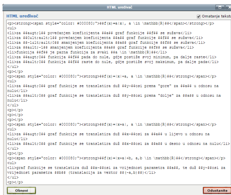
Slika 3.1: HTML uređivač
