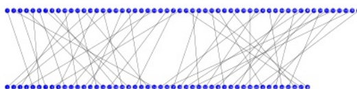
Slika 1.7: Shema kompresijske permutacije PC2
