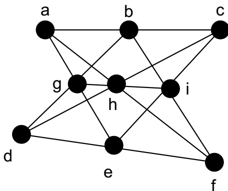
Slika 11: Slika Pappusovog matroida.
