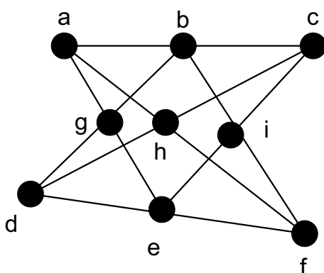
Slika 12: Slika ne-Pappusovog matroida.
