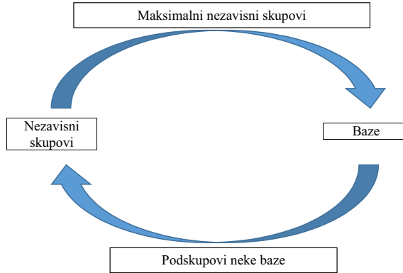
Slika 25: Kriptomorfizam između nezavisnih skupova i baza.
