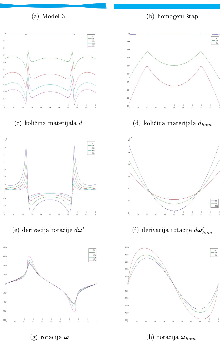
Slika 4.14: Usporedba rezultata numeričkih simulacija za Model 3 i odgovarajući homogeni štap
