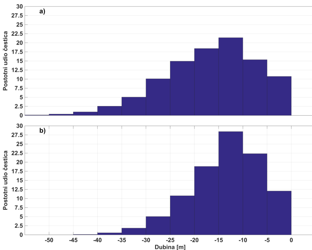
Slika 23. Raspodjela čestica po dubinama u simulaciji unazad na dane 17. srpnja (a) i 5. kolovoza 2011. godine (b) nakon što je 20000 čestica ispušteno južno od otoka Mljeta 1. rujna u pokusu 1. (tablica 4).
