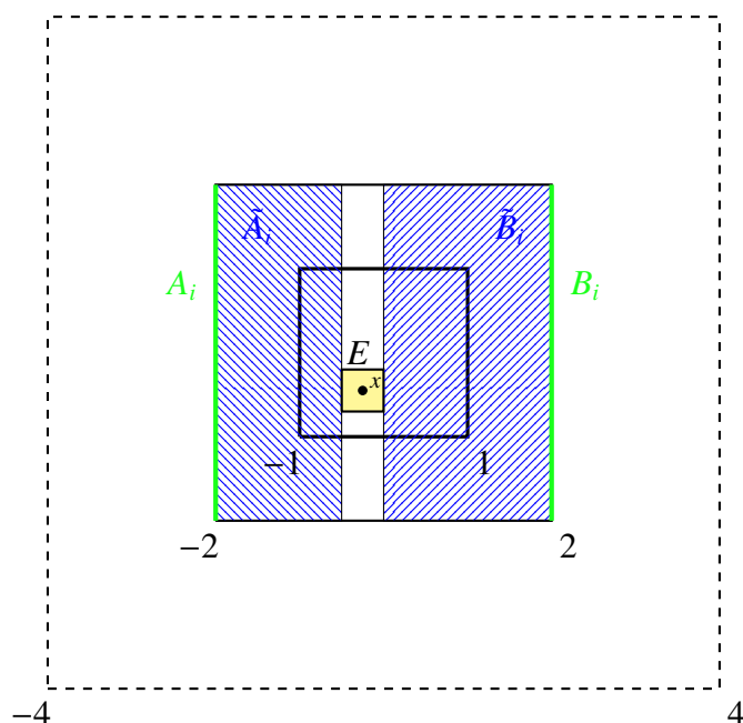
Slika 3.2: Vizualizacija dokaza.
