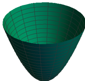
Slika 1.15: Rotacijski paraboloid
