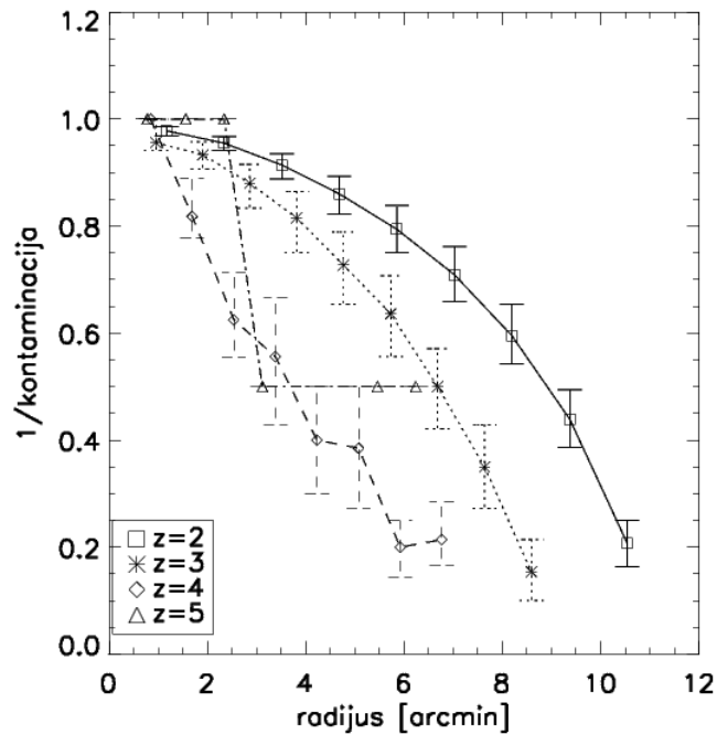
Slika 15: Ponašanje kontaminacije za protojata u ovisnosti o udaljenosti od središta, na crvenim pomacima z=2, 3, 4 i 5 . Prikazane funkcije su vrijednosti medijana i interkvartilni rasponi kontaminacija za 1000 simuliranih protojata (za svaki tip protojata na svakom crvenom pomaku). Ponašanje funkcija kontaminacije je prikazano funkcijom n_{kont}^{-1} radi lakše vizualizacije.
