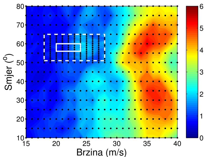
Slika 3.2: Maksimalna valna visina (m) na vrhu Zaljeva Vela Luka na Korčuli u ovisnosti o brzini ( x os) i smjeru ( y os) propagacije poremećaja tlaka zraka. Bijeli pravokutnici označavaju raspon brzina i smjerova koji odgovaraju poremećaju zabilježenom 21. lipnja 1978. godine - punom linijom označen je raspon određen u Orličevom radu iz 1980. [24], a crtkanom linijom raspon dobiven u radu Orlića i sur. iz 2010. [12] u kojem se pretpostavilo da je vremenska greška barografskih zapisa bila \pm 10 min. Crne točke označavaju simulacije.
