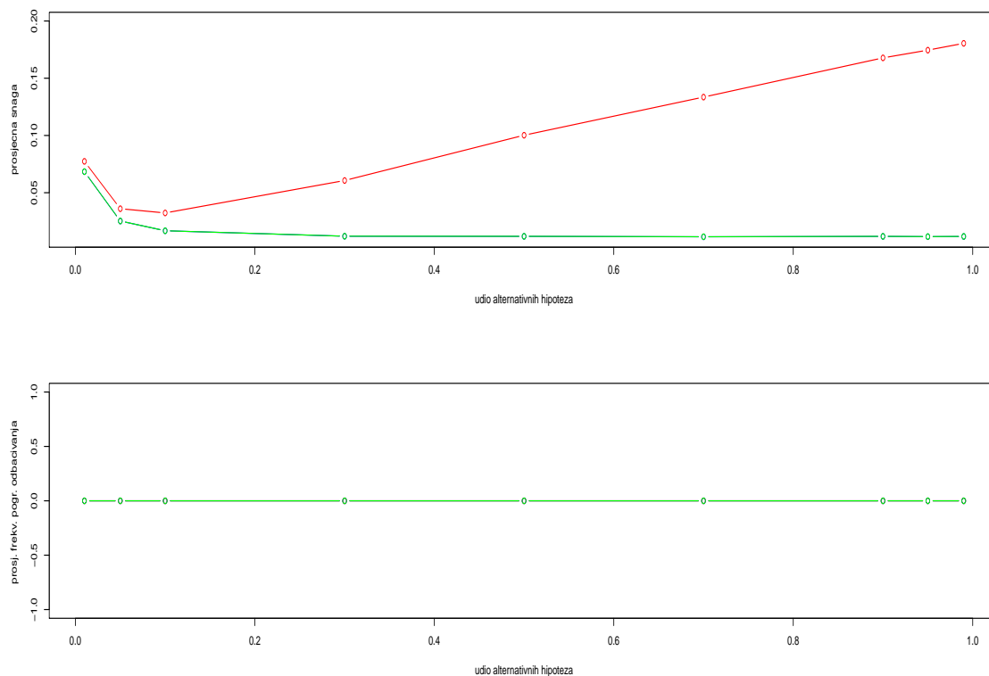
Slika 3.1: prosječna snaga i prosječna frekvencija pogrešno odbacjenih nul hipoteza za q^* = 0.01 , odnosno \alpha = 0.01 (crvena linija \leftrightarrow FDR, zelena linija \leftrightarrow Holm's i FWER)
