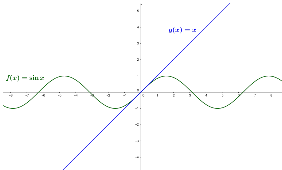
Slika 1.1: Taylorov polinom prvog stupnja za funkciju sinus
