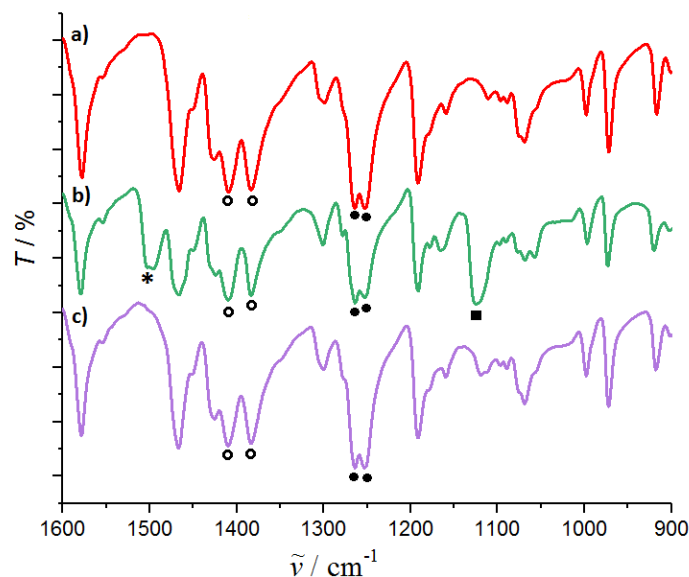
Slika 34. IR spektar spoja 2 nakon sublimacije snimljen u KBr pastili a) prije ozračivanja UV svjetlom pri 14 K; b) nakon ozračivanja 2 sata UV svjetlom pri 14 K; c) nakon zagrijavanja na 298 K. Karakteristične vrpce asimetričnog i simetričnog istežanja Z -azodioksidne veze označene su šupljim crnim kružićem (○), vrpce asimetričnog istežanja E -azodioksidne veze označene su punim crnim kružićem (●), dok su vrpce istežanja N=O i C–N veze monomera označene zvjezdicom (*), odnosno kvadratićem (■)
