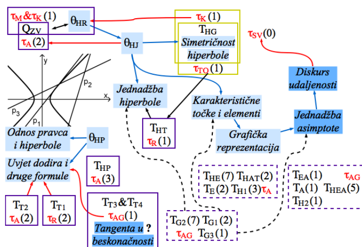
Slika 5.2.11: Grafički prikaz prakseološke organizacije jedinica unutar teme Krivulje drugog reda u udžbeniku drugog seta
