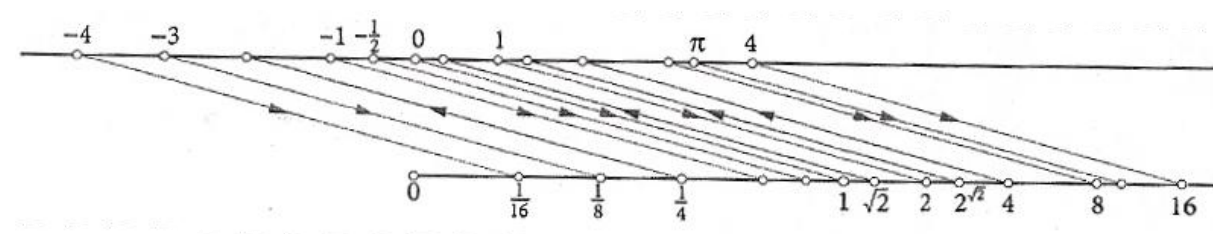
Slika 5.2.7: Tehnika pridruživanja točaka domene točkama kodomene iz udžbenika drugog seta
