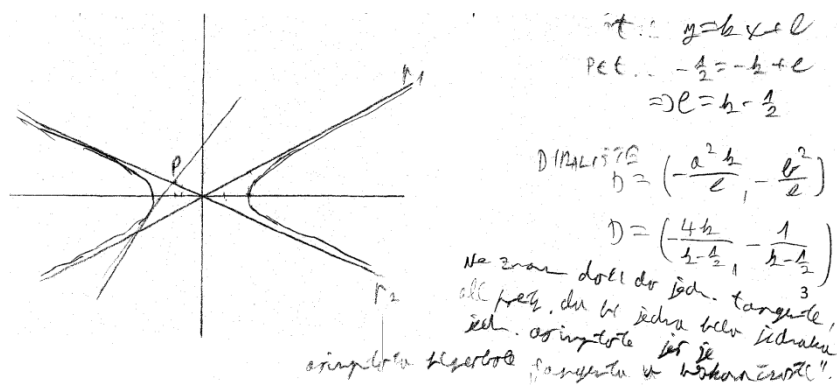
Slika 5.3.24: Hiperbola iz praxisa P_{TA} i pogrešno prikazanim pravcem kroz točku P zbog nedostatka odgovarajućeg praxisa , ali s poznavanjem ispravnog logosa u odgovoru na Pitanje 3.3
