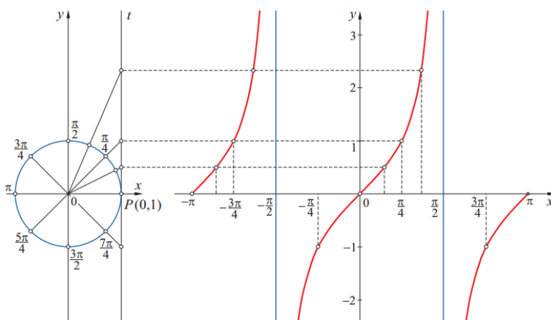
Slika 5.2.2: Tehnika konstrukcije ordinata točaka funkcije tangens prenošenjem odgovarajućih duljina s brojevnice iz udžbenika prvog seta
