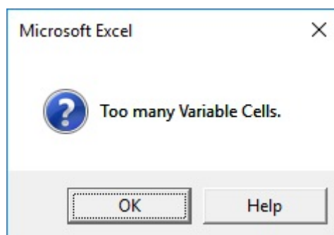
SLIKA 4.2. Solver poruka.
