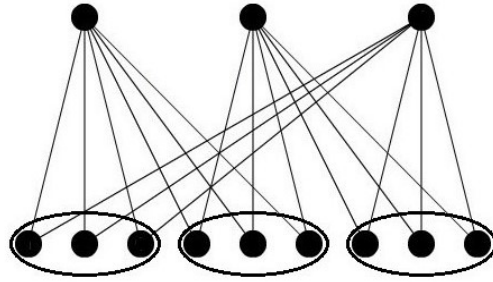
Slika 2.4: Incidencijska struktura tranzitivna po incidencijama
