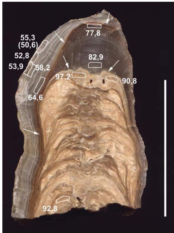
Slika 3: Potopljena siga iz jame U vode na otoku Krku. Odredba starosti sige napravljena je metodom U-Th (pravokutnici), a dobiveni rezultati su dani u tisućama godina prije sadašnjosti (preuzeto iz Surić, 2006).
