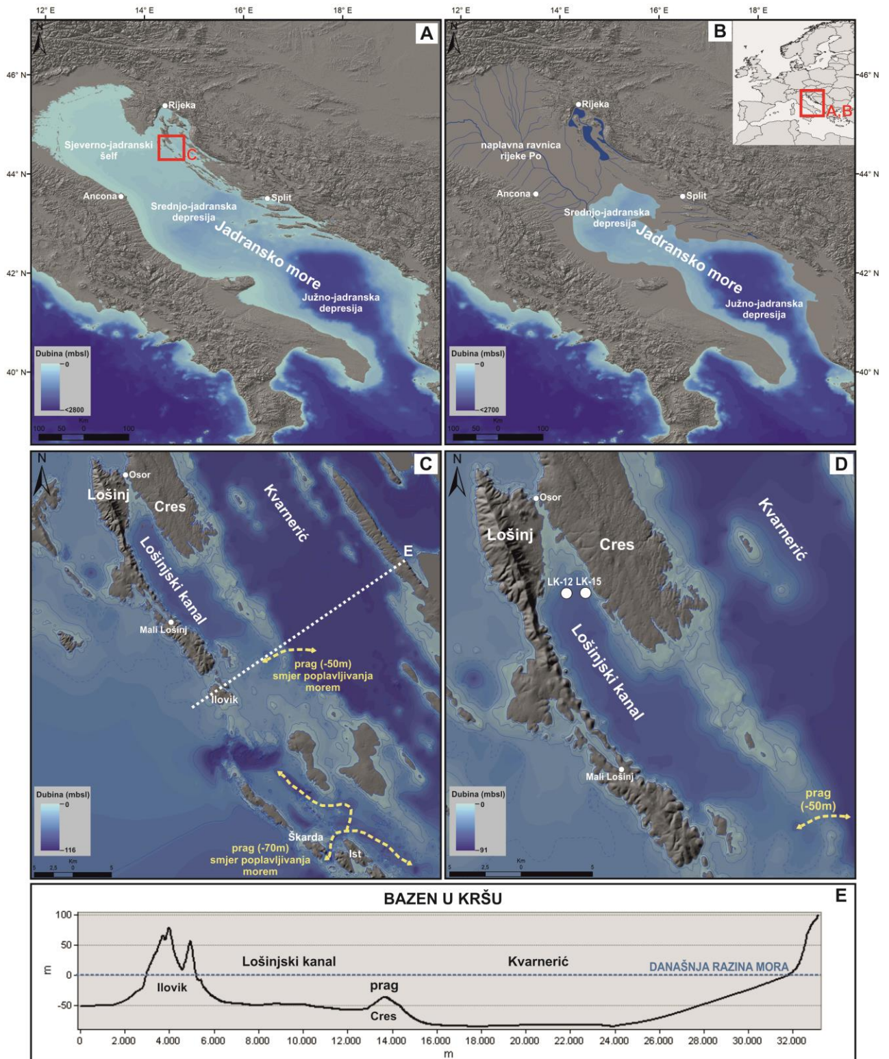
Slika 10: Batimetrijske karte i poprečni presjek istraživanog prostora: A) batimetrijska karta Jadranskog mora, B) Jadransko more tijekom LGM-a (zapadna obala Jadrana modificirana je prema Maselli et al., 2011; Maselli & Trincardi, 2013; istočna obala Jadrana modificirana je koristeći batimetrijske podatke (Becker et al., 2009), te podatke iz Sikora et al., 2014 i Miko et al., 2016), C) batimetrijska karta Lošinjskoga kanala s naznačenom lokacijom praga i smjerom intruzije mora (žuta strelica), D) batimetrijska karta Lošinjskoga kanala i lokacije bušenja jezgara sedimenata LK-12 i LK-15, E) poprečni presjek Lošinjskoga kanala. Lokacija poprečnog presjeka označena je na karti C.
