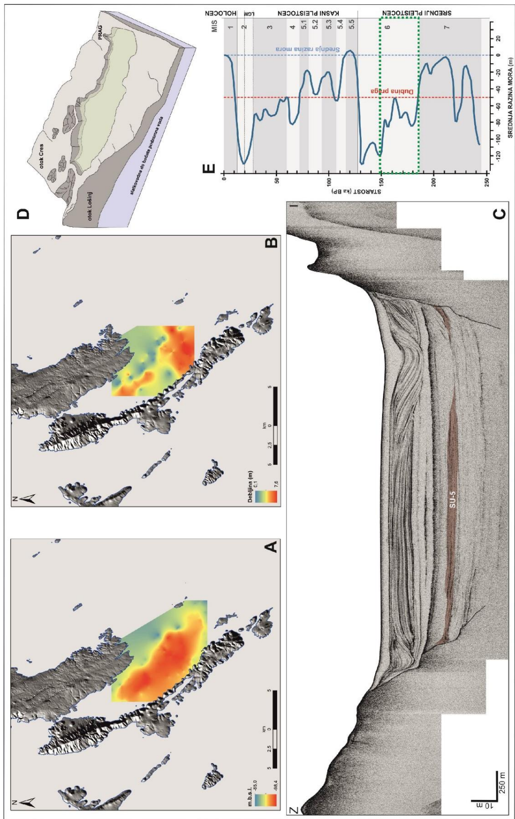
Slika 119: Lošinjski bazen u kršu: A) karta reflektora baze jedinice SU-5, B) karta debljine sedimenata, C) seizmički profil visoke rezolucije s označenom seizmičkom jedinicom SU-5, D) rekonstruirani paleookoliš, E) krivulja promjene morske razine (modificirano prema Waelbroeck et al., 2002) s označenim vremenskim trajanjem taloženja sedimenata jedinice (zeleni pravokutnik).
