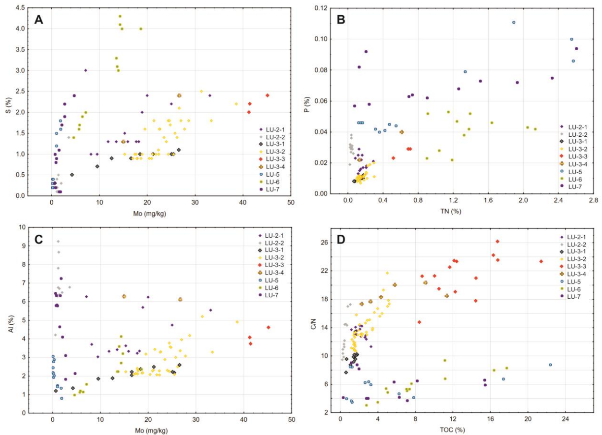
Slika 144: Dijagrami rasprišenja elemenata u jezgrama LK-5, LK-6 i LK-7, te izdvojenim jedinicama jezgara LK-2 i LK-3. A) S-Mo, B) N-P, C) Mo-Al, D) TOC-C/N.
