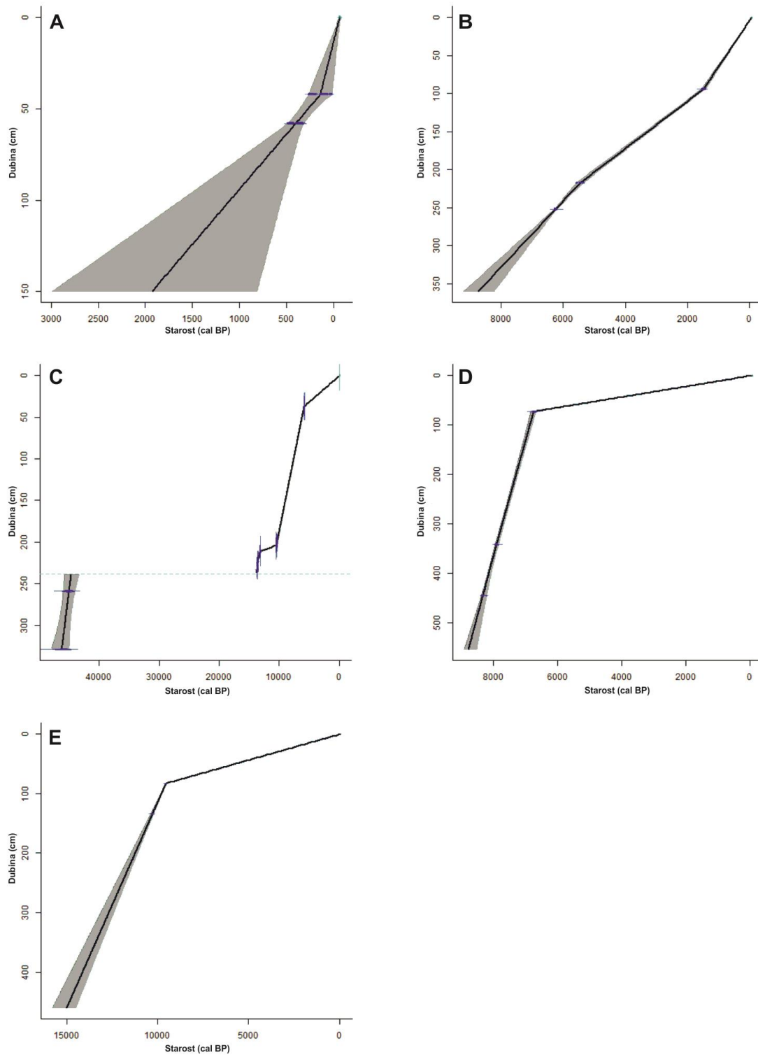
Slika 34: Model dubina-starost za jezgre sedimenata: A) LK-2, B) LK-3, C) LK-12, D) LK-13, E) LK-15. Rezultati datiranja metodom radioaktivnog ugljika ( AMS^{14}C ) linearno su interpolirani s primjenjenom korekcijom na rezervoar efekt. Plave oznake na slici označavaju dobivene rezultate datiranja. Sivo osjenčano područje označava raspon vjerojatnosti rezultata.
