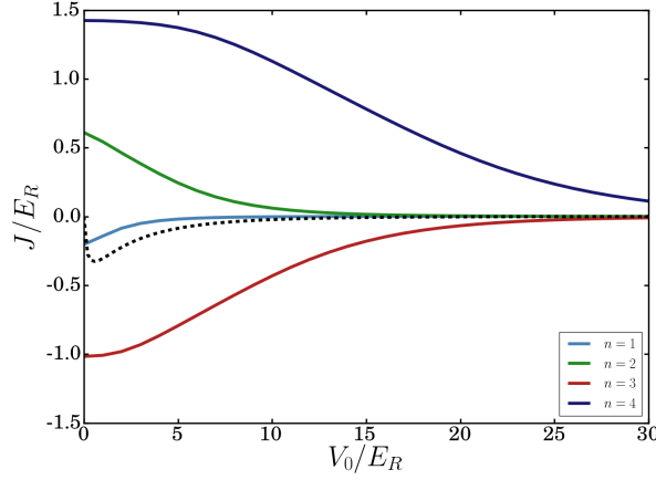
Slika 3.4: Parametar preskakanja između prvih susjeda za četiri najniže energijske vrpce u jedinicama E_R = \hbar^2 \pi^2 / 2ma^2 za potencijal V(x) = V_0 \cos(kx) . Crnom crtkanom linijom je prikazan parametar preskakanja za najnižu vrpcu prema jednačbi (3.25).
