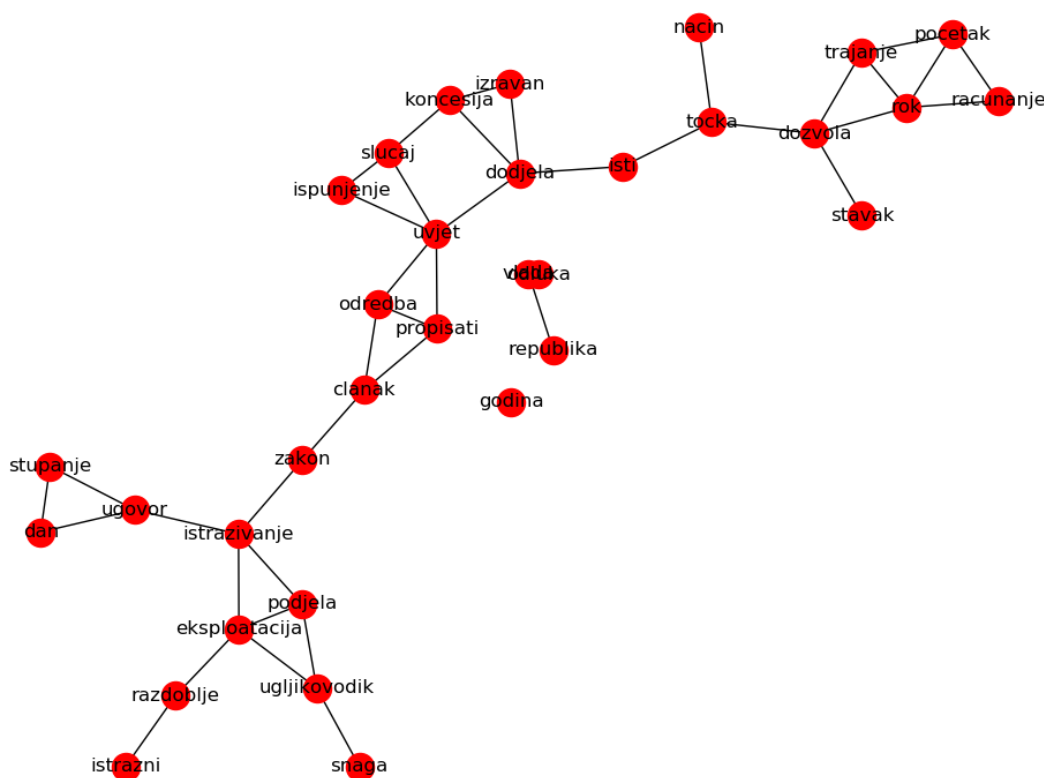
Slika 3.1: Konstruirani graf
