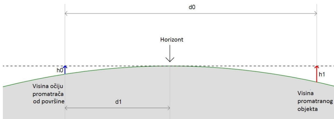
Slika 1.1 Zakrivljenost Zemlje
