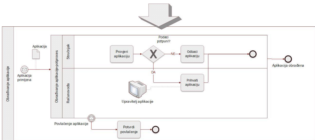
Slika 3.2. Pretvorba UML modela u BPMN model
