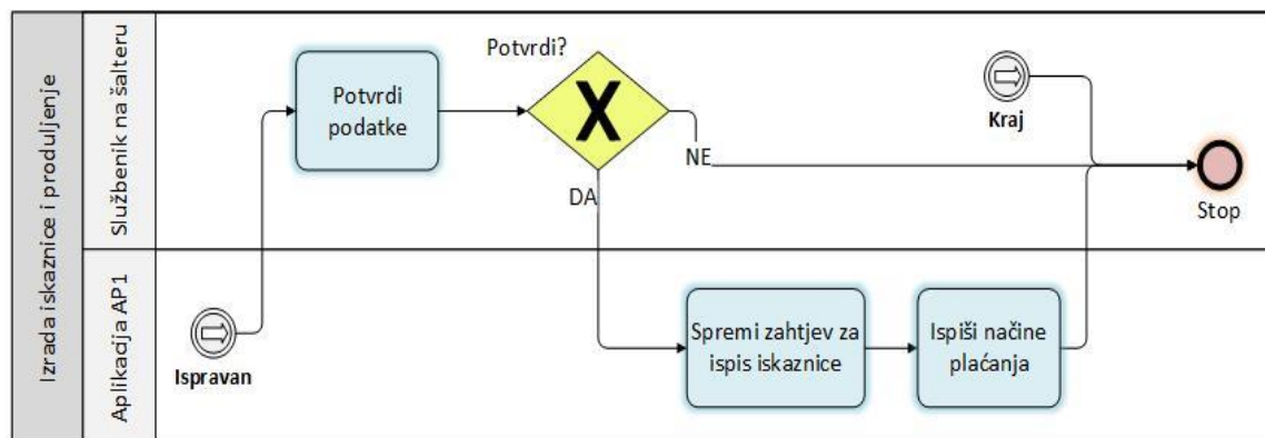
Slika 4.8. Potproces „Izrada iskaznice i produljenje“, drugi dio
