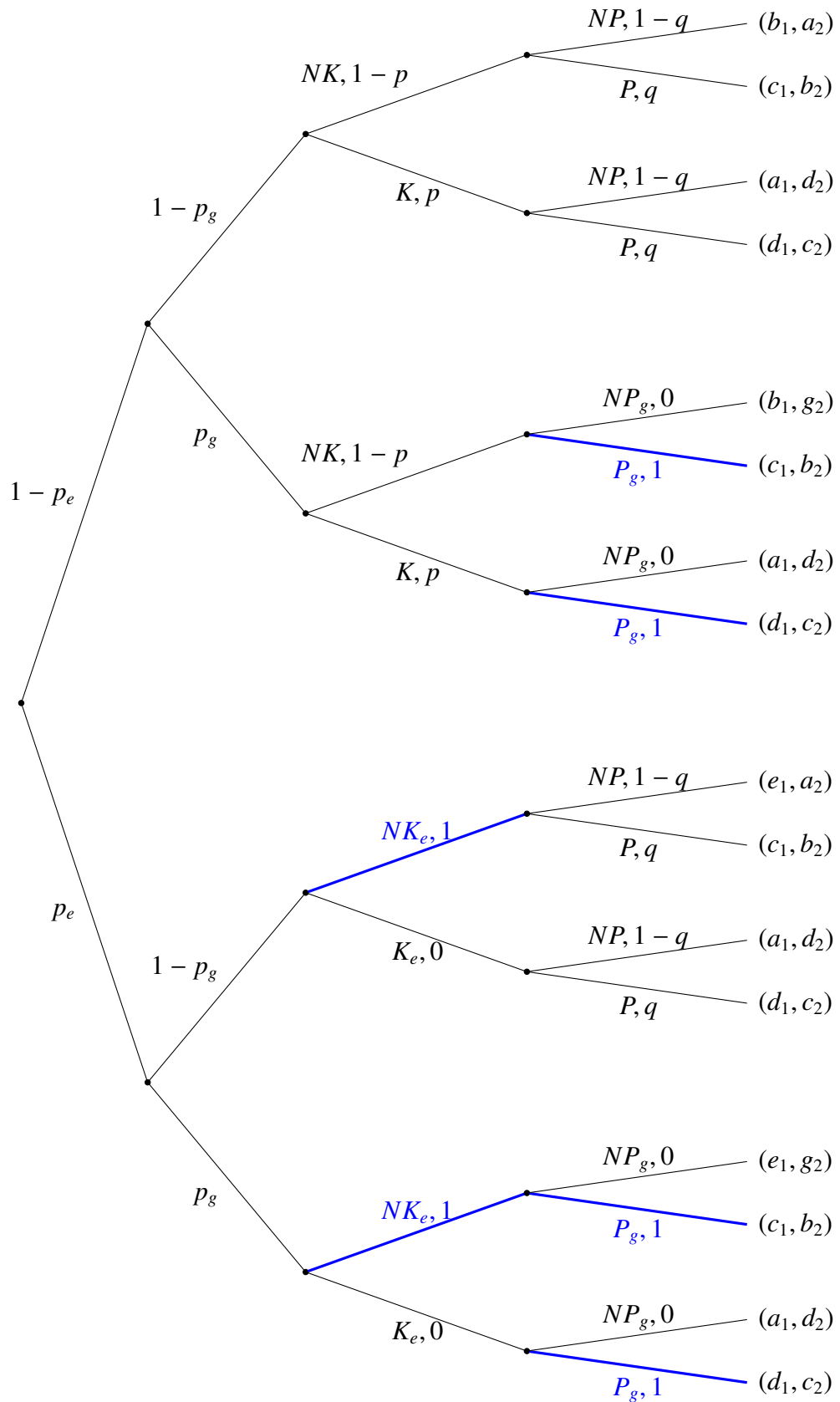
Slika 2.1: Stablo 1
